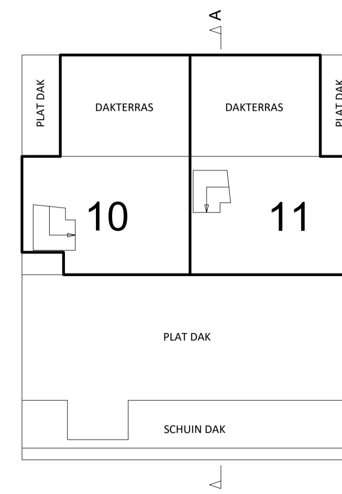
5E VERDIEPING 1:100
