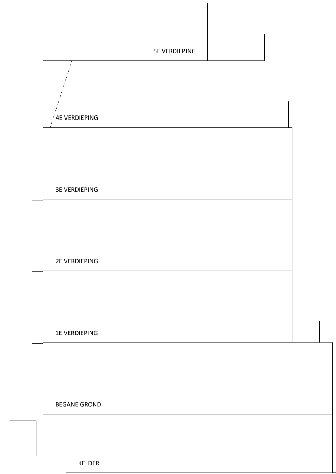
DOORSNEDE A-A 1:100
