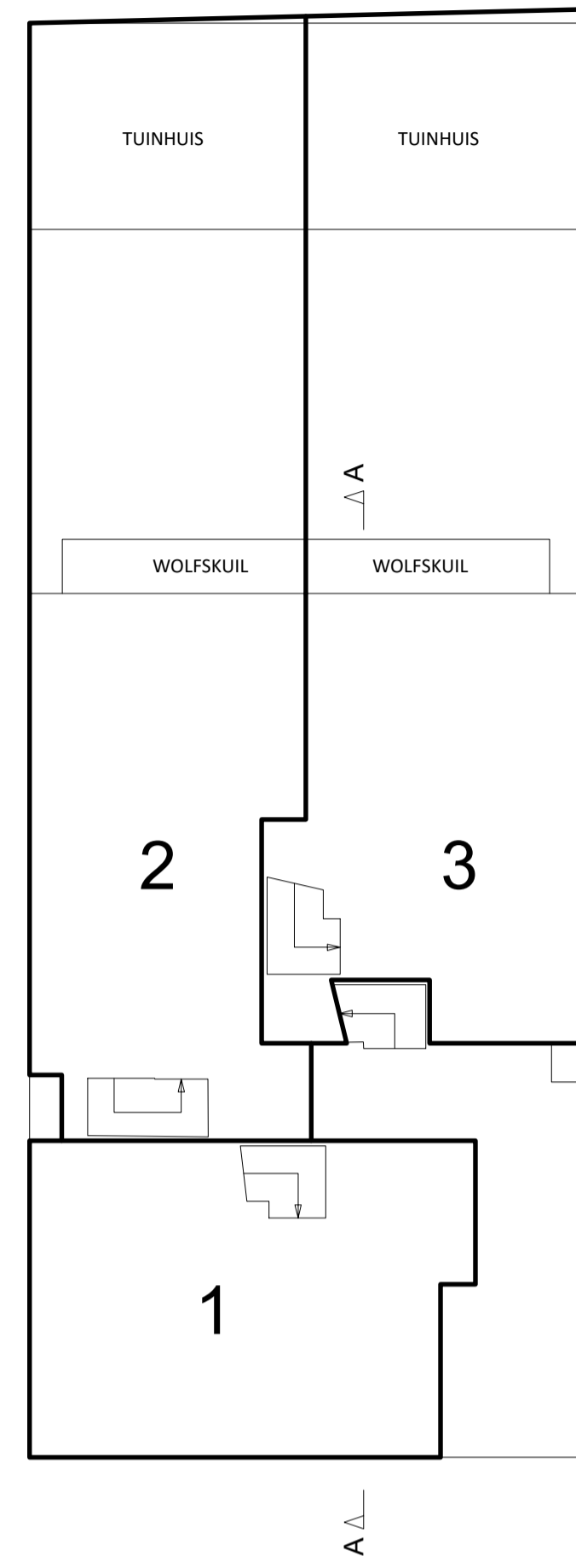
BEGANE GROND 1:100
